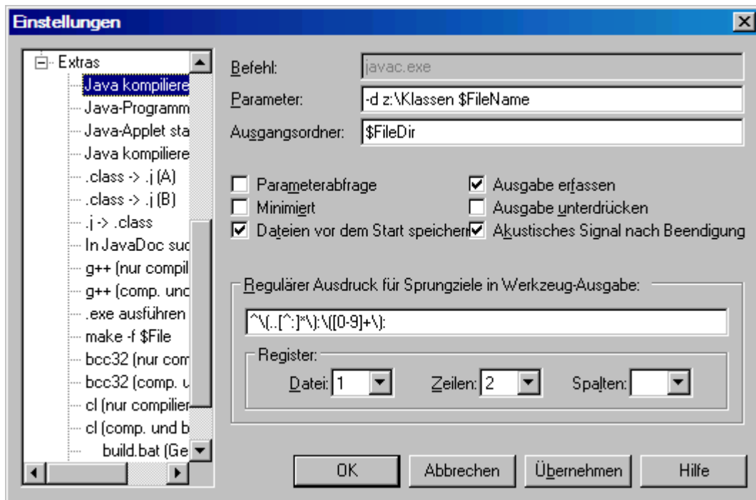
Abb. 5: Einstellungen für den Befehl Java kompilieren
